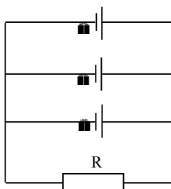
Рис. 2.3. Схема электрической цепи к задаче 2.34
