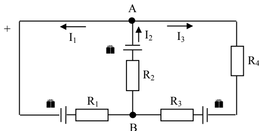
Рис. 2.2. Электрическая цепь
